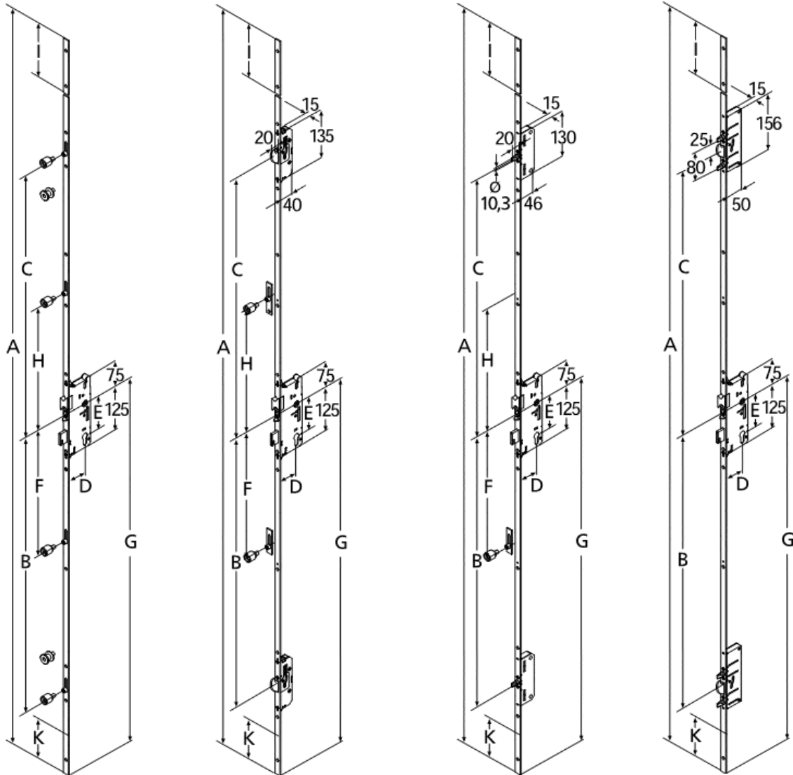
Maße/dimensions Typ 1 + 2
