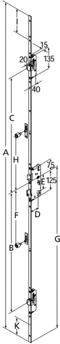
Maße/dimensions Typ 1 + 2
