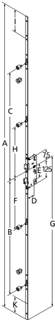
Maße/dimensions Typ 1 + 2
