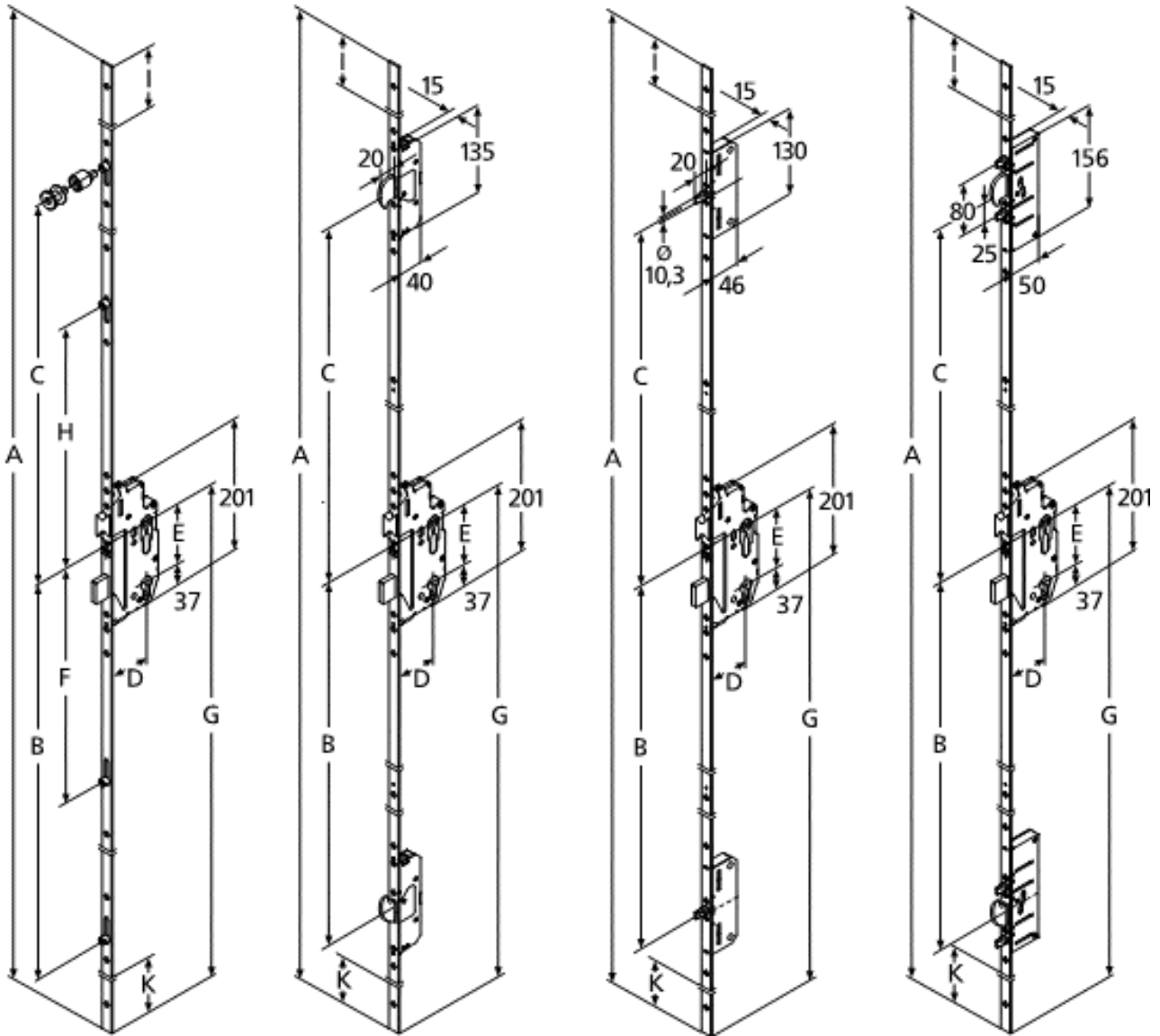
Typ 1 + 2
